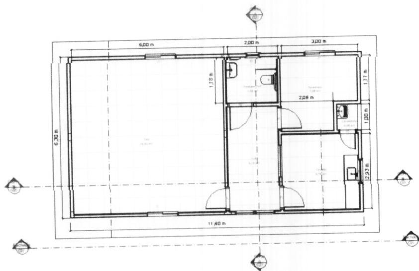
Imagem 02. Projeto arquitetônico – Planta Baixa – reprogramado do projeto com área construída de 73,08m 2 ; projeto arquitetônico com as devidas alterações e dimensionamento.
